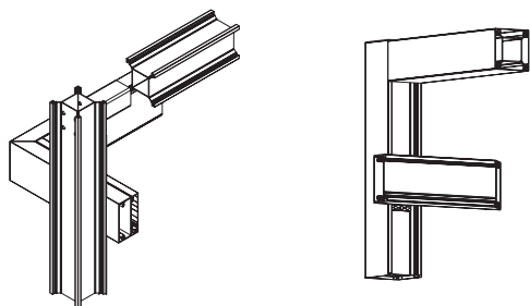
Σύνδεση προφίλ κολόνας και τραβέρσας
