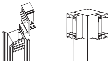
Σύνδεση κολόνας με τραβέρσα
