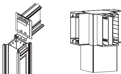
Σύνδεση κολόνας με ενδιάμεση τραβέρσα
